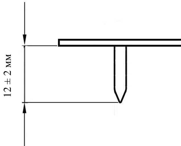
Рисунок Д2.1 – Розміри штифта (гвіздка)
