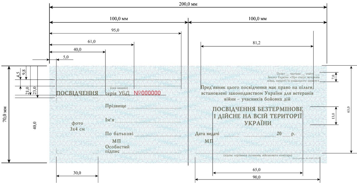
Рисунок 2 – Зовнішній вигляд та лінійні розміри внутрішньої частини предмета у розгорнутому вигляді
