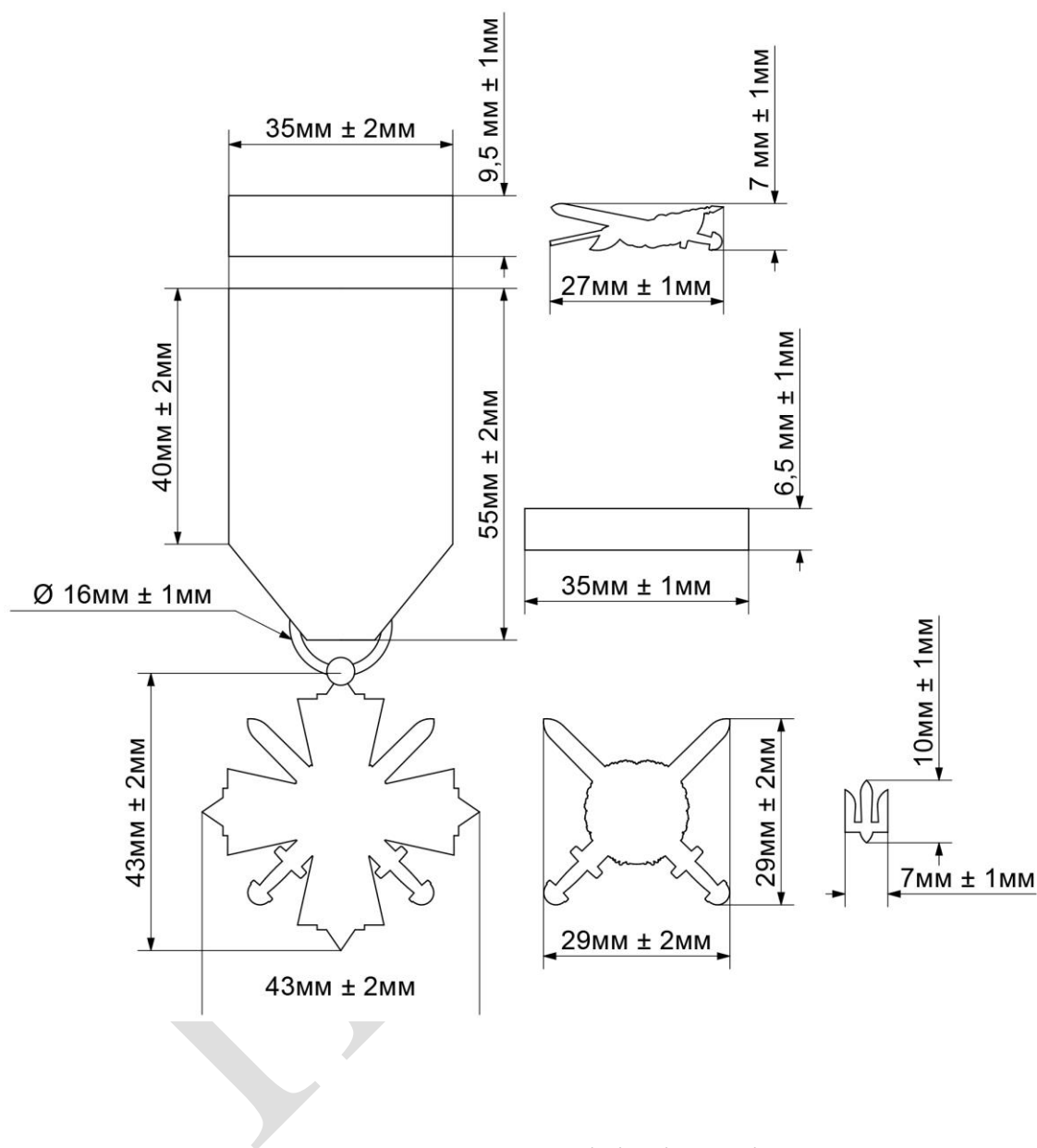
Рисунок 2 – Лінійні розміри предмета
