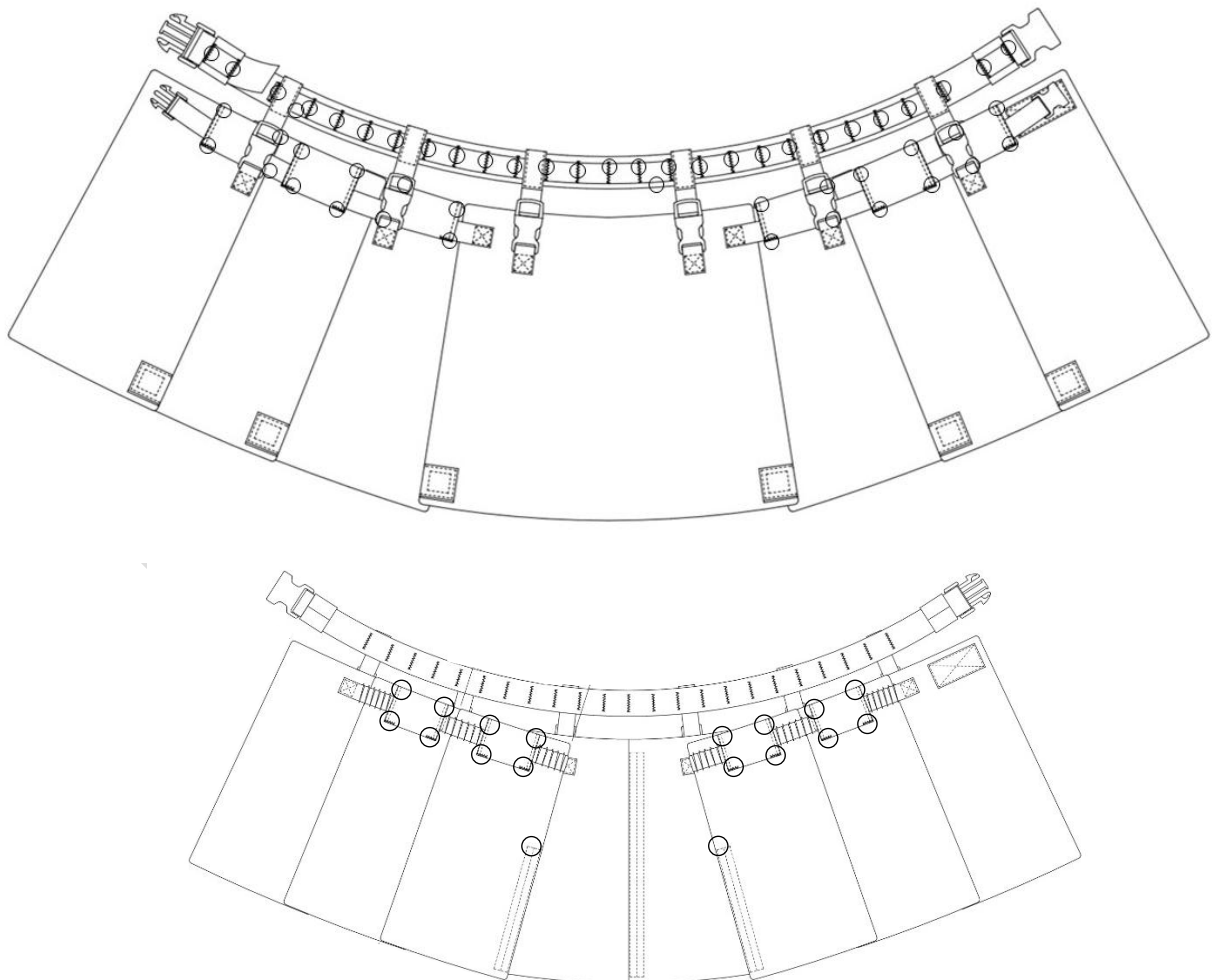
Рисунок Д5.3 – Орієнтовні місця розташування закріпок елемента 3 (примітка: закріпки розташовуються по верху входів всіх передніх та бокових клинів)
