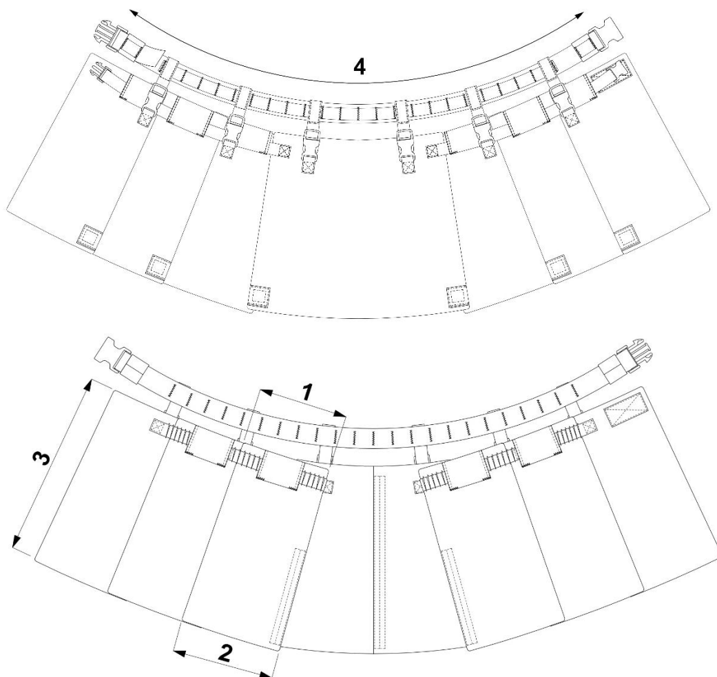
Рисунок Д2.3. – Орієнтовне позначення лінійних вимірів елемента 3
