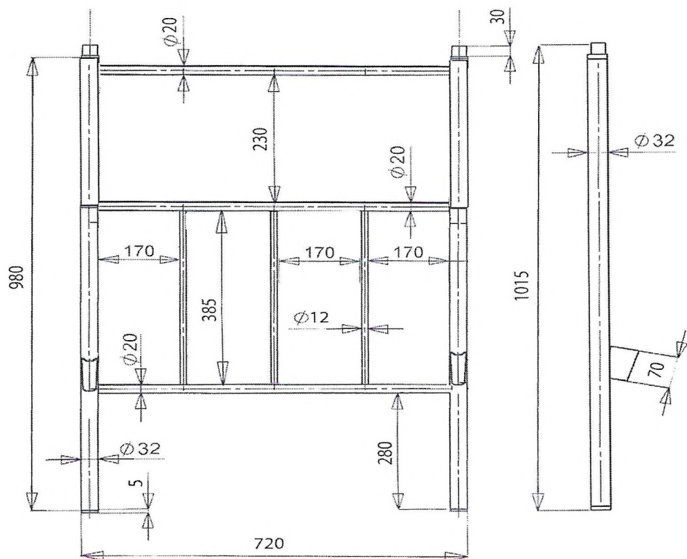
Мал. 5. Зовнішній вигляд верхньої спинки ліжка двоярусного розбірного ЛДР-Т1
