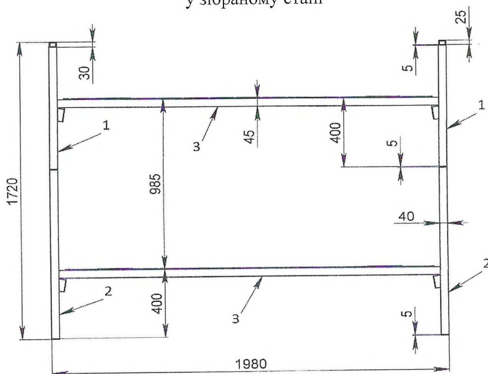
Мал.1. Зовнішній вигляд ліжка двоярусного розбірного ЛДР-Т2 у зібраному стані
