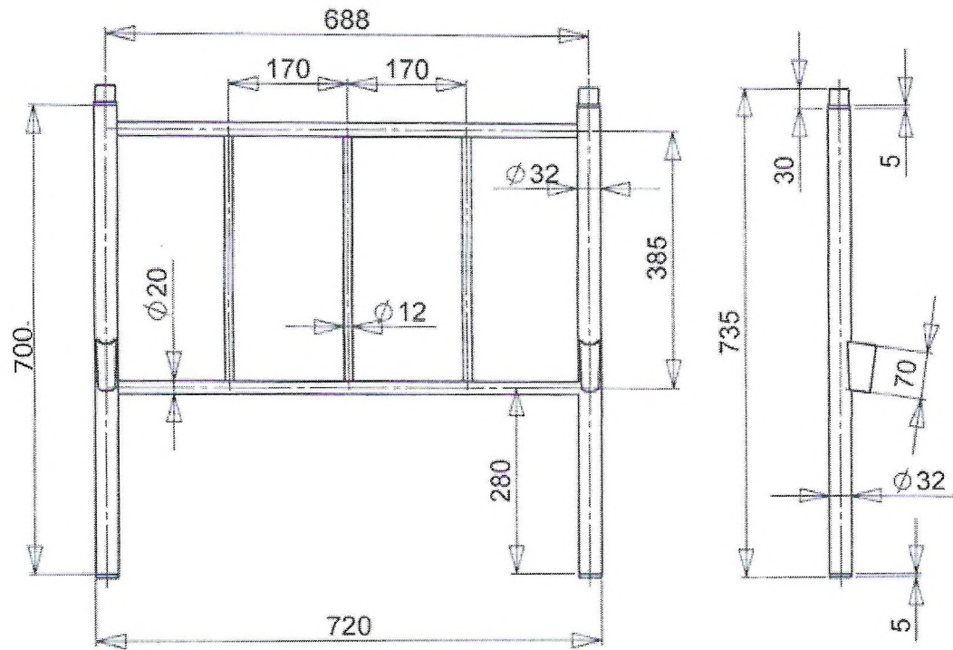
Мал. 5. Зовнішній вигляд верхньої спинки ліжка двоярусного розбірного ЛДР-Т1
